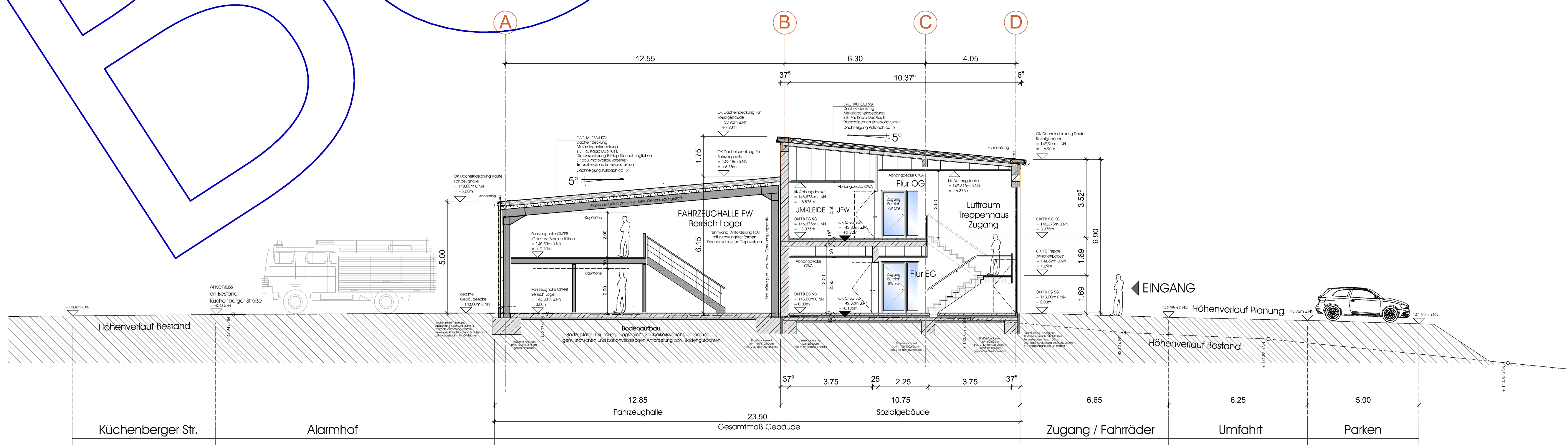
Systemschnitt C - C
